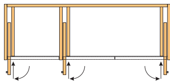
Montážní schéma pro vložené dveře
