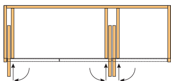
Montážní schéma pro naložené dveře s bočnicemi
