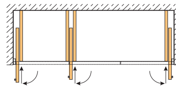
Montážní schéma pro dveře ve zdi
