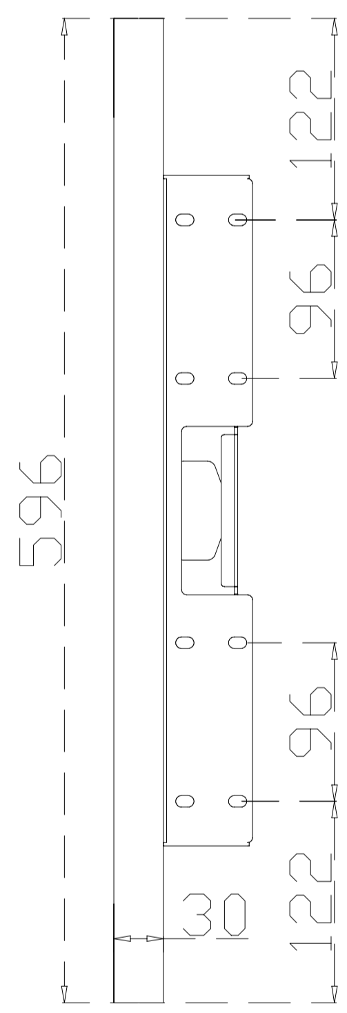
Q 7206 * 600 mm
