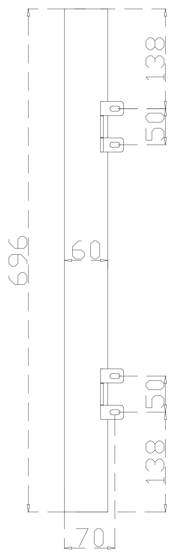
MQ 7907 * 700 mm
