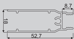
Lišta vodotěsná dolní (5000 mm) obj. 1465x
