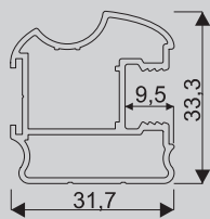
Profil Exclusive (2700 mm) obj. 1467x
