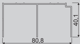
Kolej horní (5000 mm) obj. 011461x
